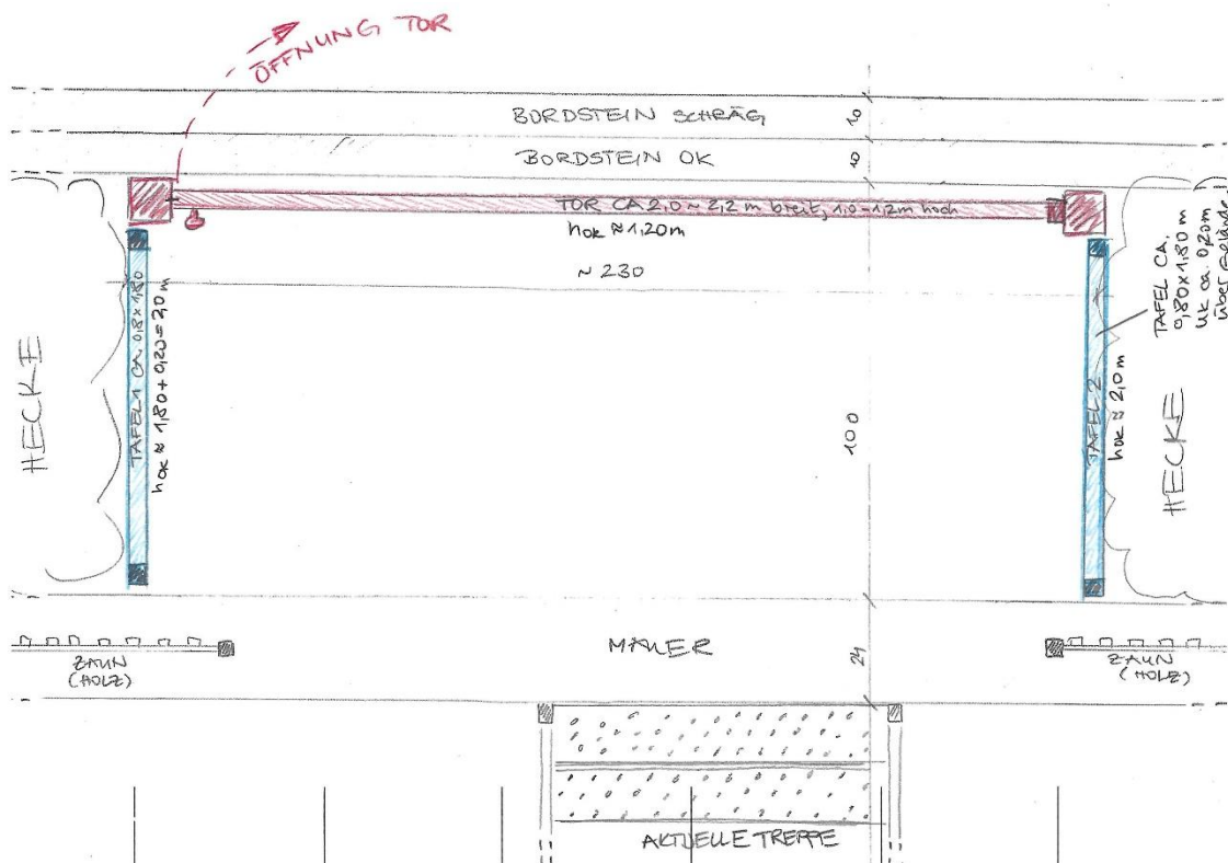
Skizze Grundriss
